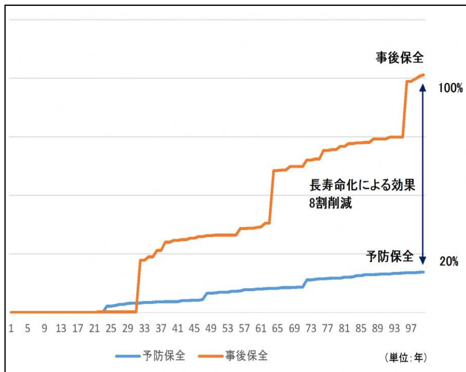
図-7 長寿命化修繕計画の効果
