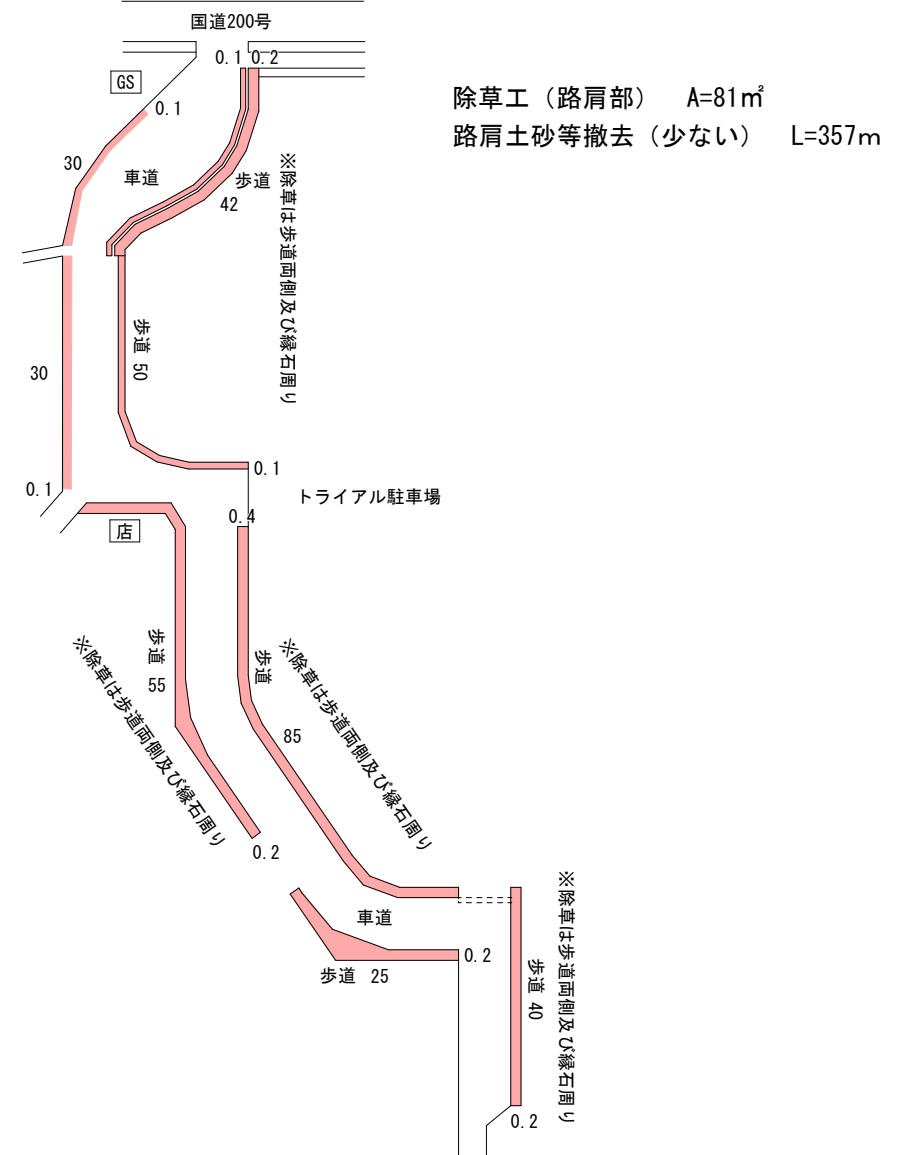
展開図（感田319号線外）
