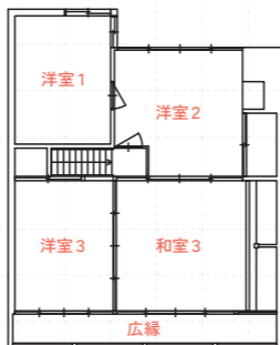
2階
