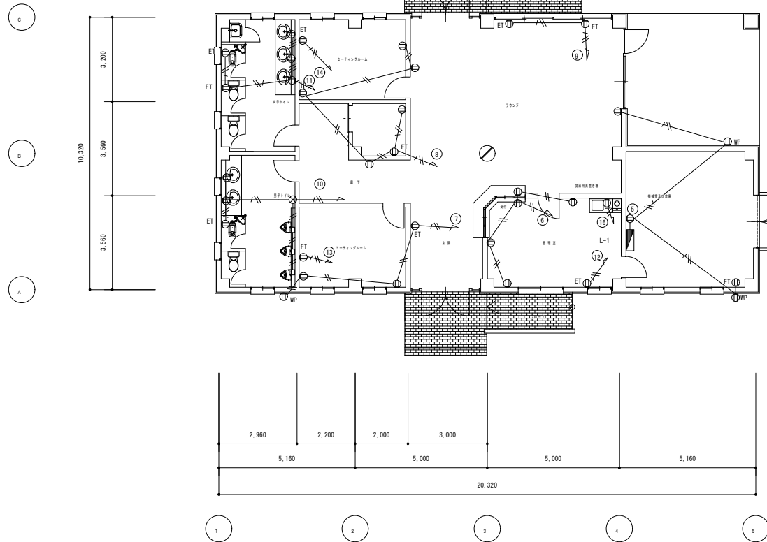
コンセント配線図 S=1:100
