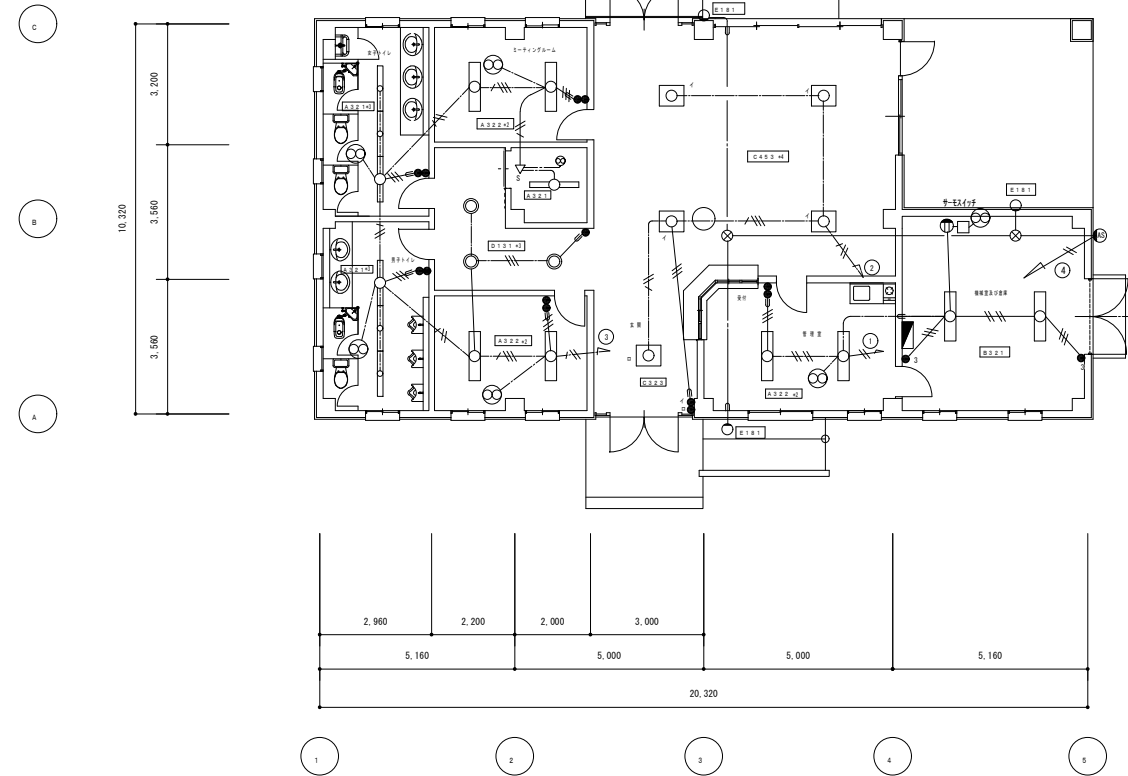
電灯配線図 S=1:100
